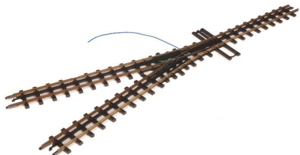
2004, 2004-L-FM und 2004-R-FM Zahnradbahnweiche
